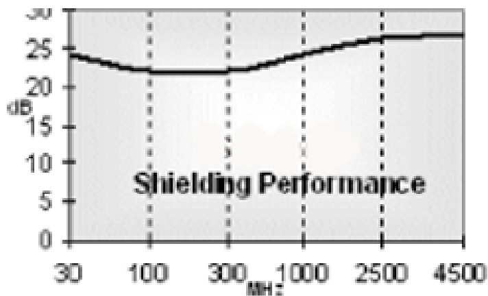
電磁波遮蔽率 vs 周波数帯グラフ
